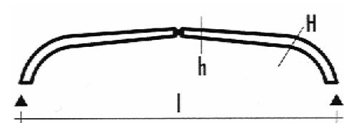
Dreigelenkrahmen mit Bogen
