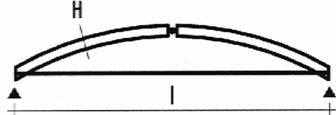
Dreigelenkrahmen mit Bogen
