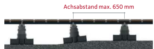
VARIO FIX mit Konstruktionsbalken 40 x 60 mm
