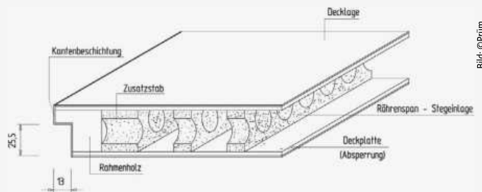
Innenleben einer Röhrenspanstreifen-tür
