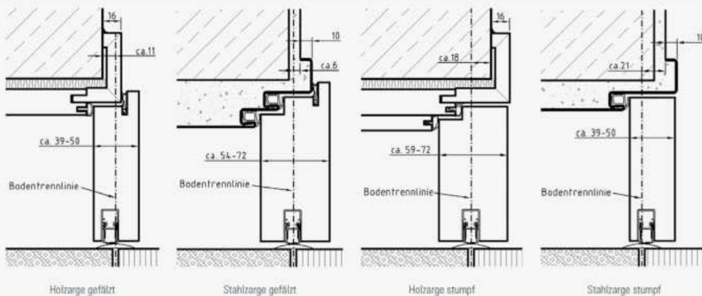
Unterschiedliche Ausführungsvarianten der Bodenschwelle
