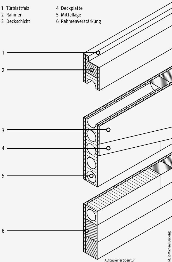
Aufbau einer Sperrtür
